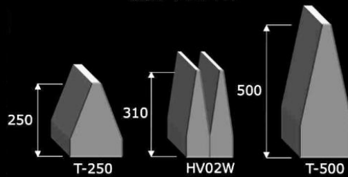
吸音クサビサイズ
