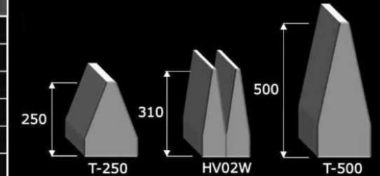
吸音クサビサイズ
